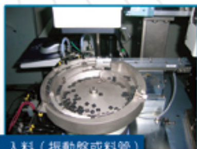
入料（振動盤或料管） Bowl/Tube feeder
